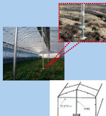
図：ハウスの補強
